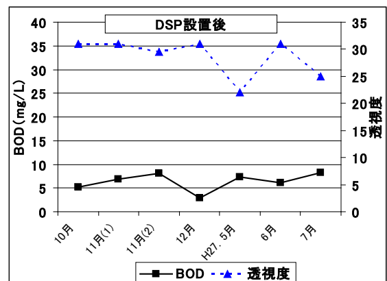
図-1 B 宅の BOD と透視度の推移
