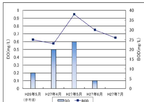
図-3 D 宅の BOD と DO の関係
