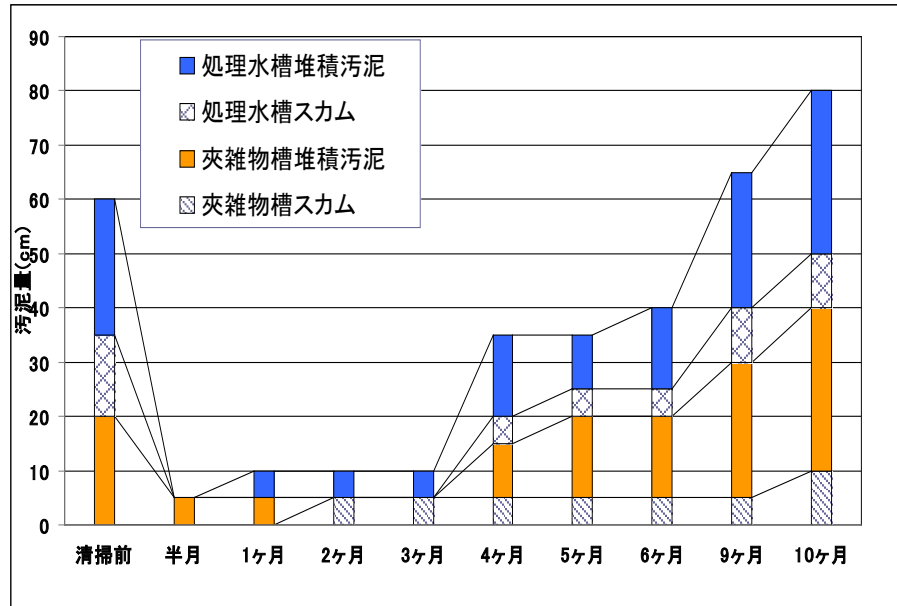
図-5 C 宅における汚泥スカム量の推移
