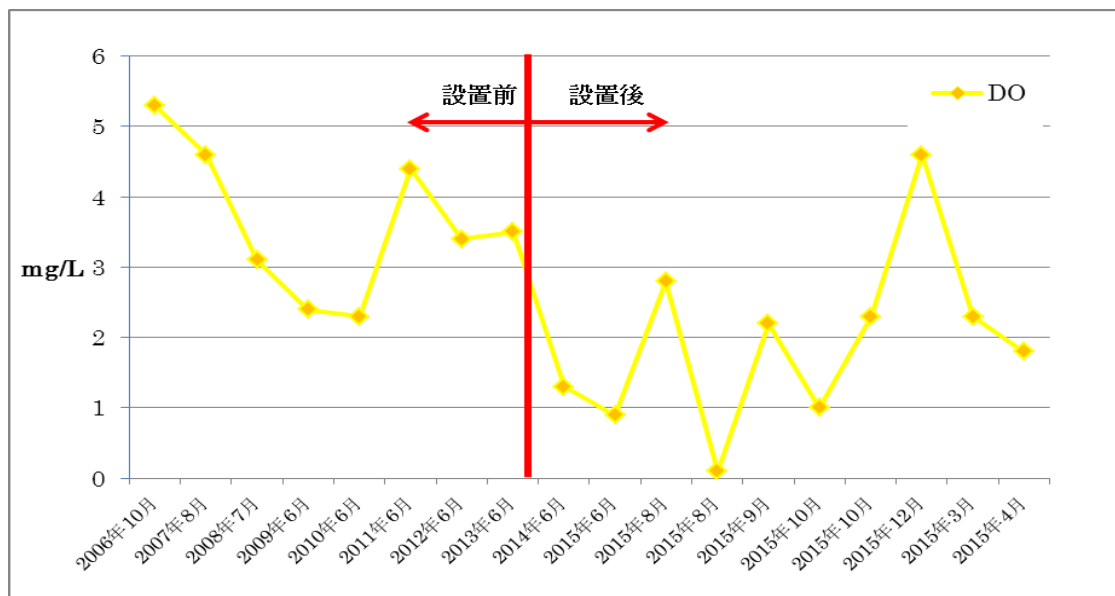
図-4 C 宅の DO の推移
