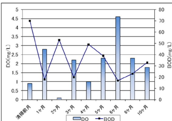
図-2 C 宅の BOD と DO の関係
